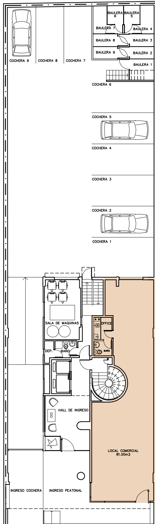
PLANTA BAJA
