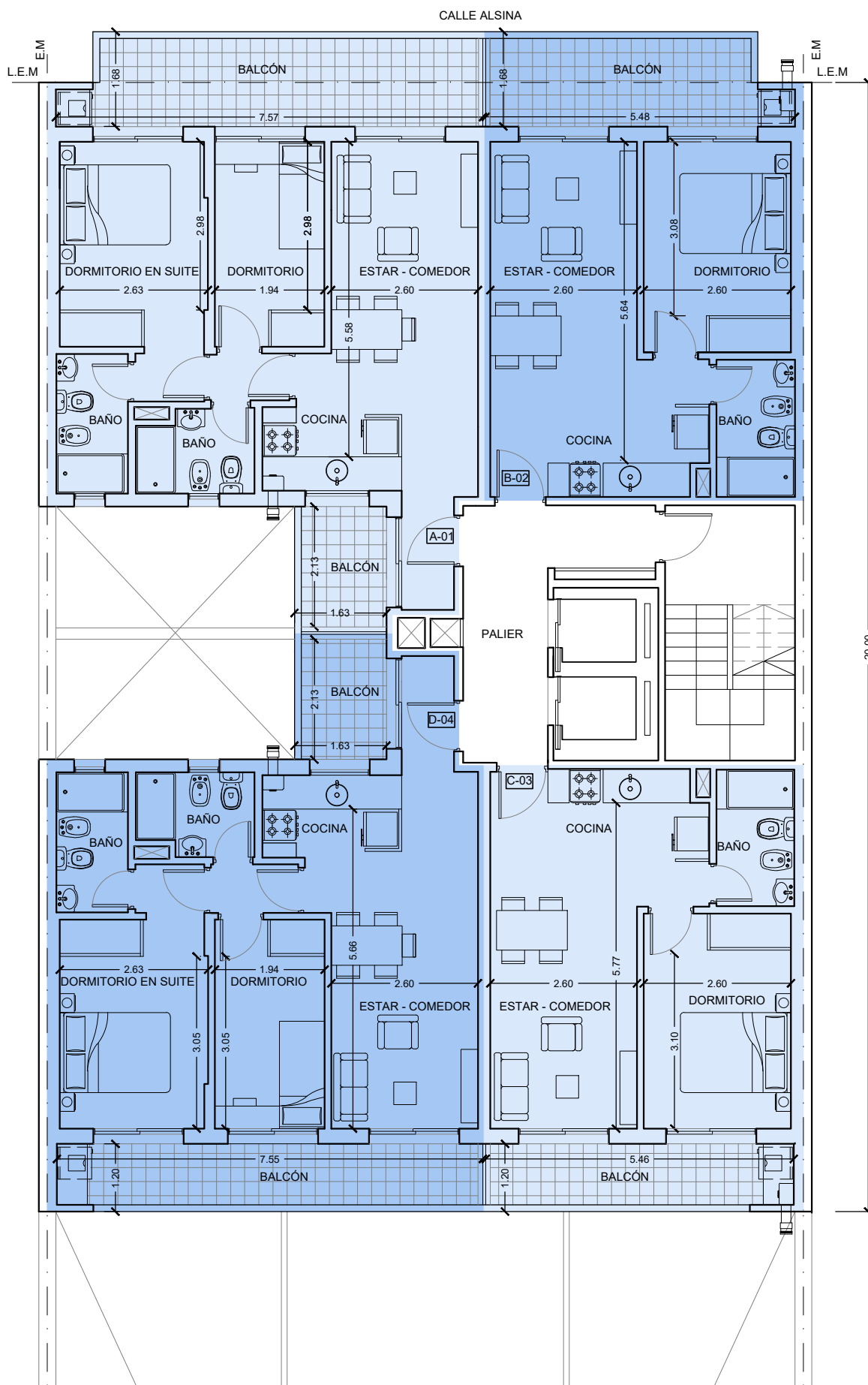
ALSINA 772 PLANTA TIPO 2º A 10º PISO
